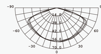
Beam angle: 148°
