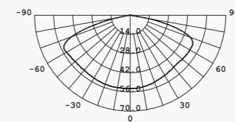
Beam angle: 148°
